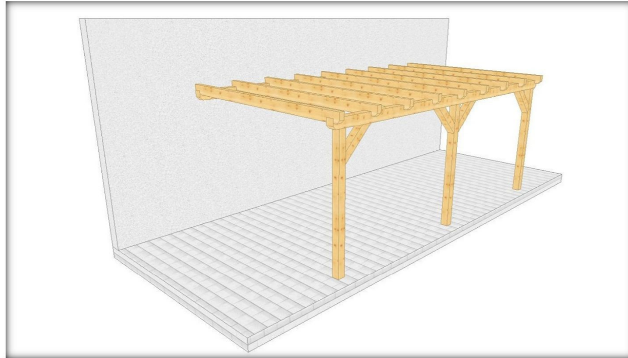
001 3 Einzelcarport
