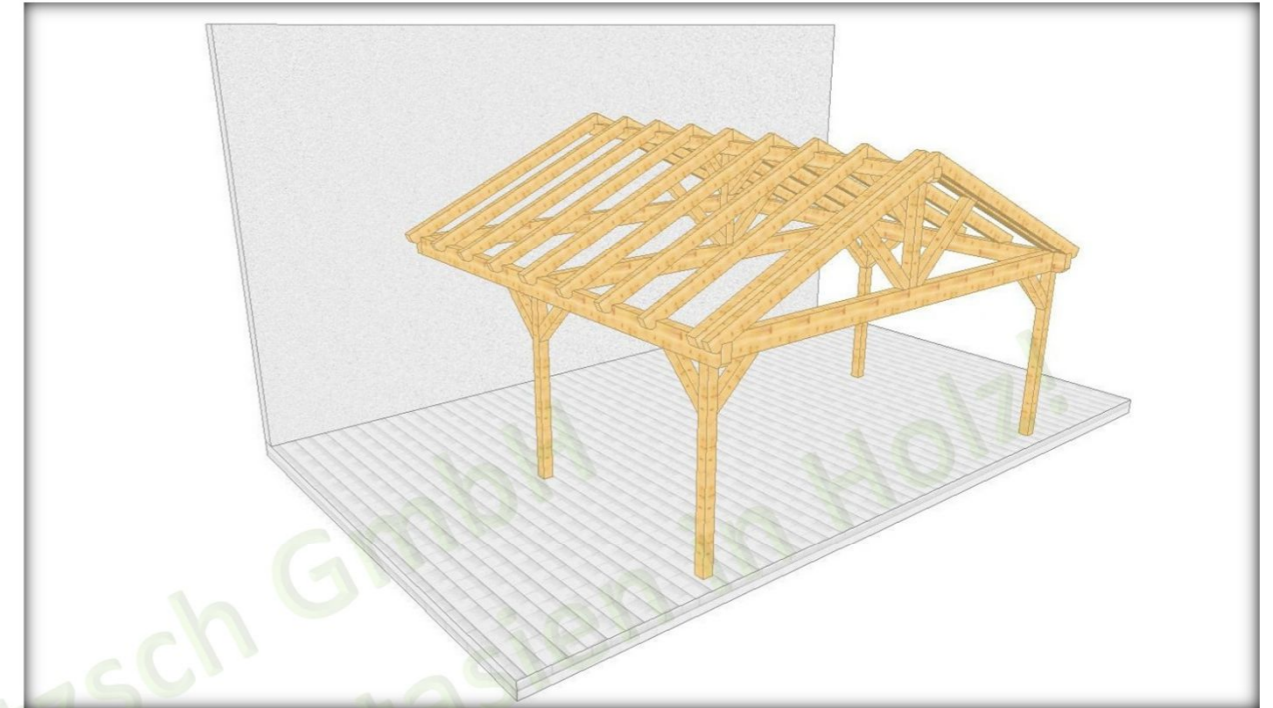
001 3 Doppelcarport
