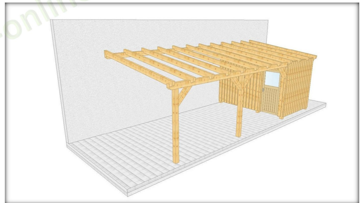
004 3 Einzelcarport mit Schuppen hinten
