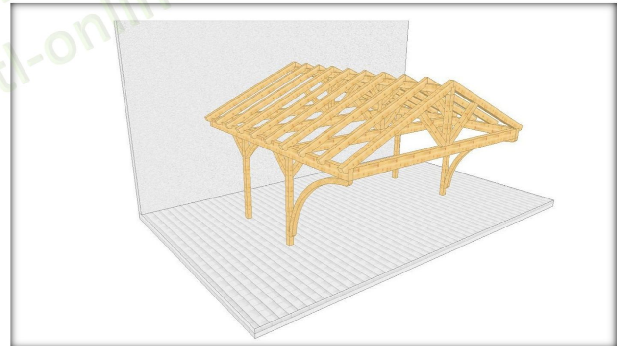
003 3 Doppelcarport mit Bogenstützen
