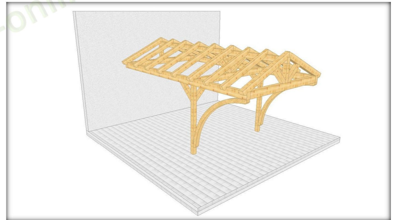
003 3 Einzelcarport mit Bogenstützen
