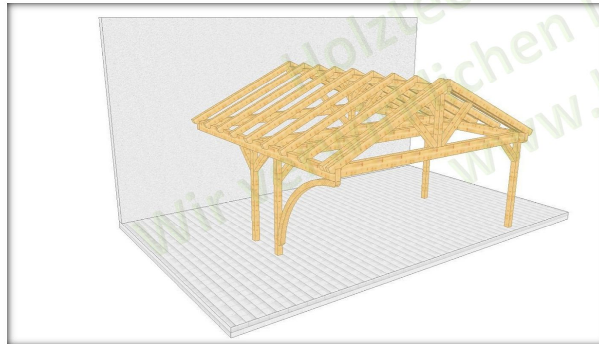
002 3 Doppelcarport mit Bogenstütze einseitig
