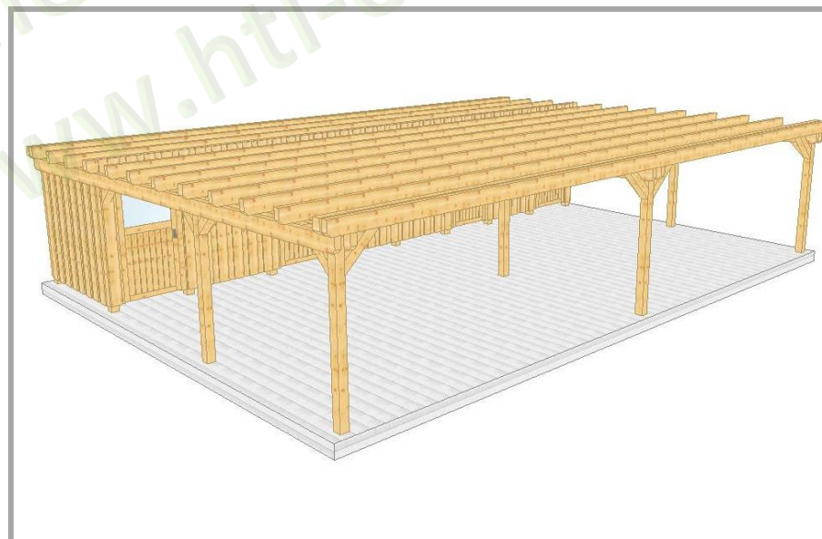
004 3 Vierfach Carport mit Flachdach und Abstellraum
