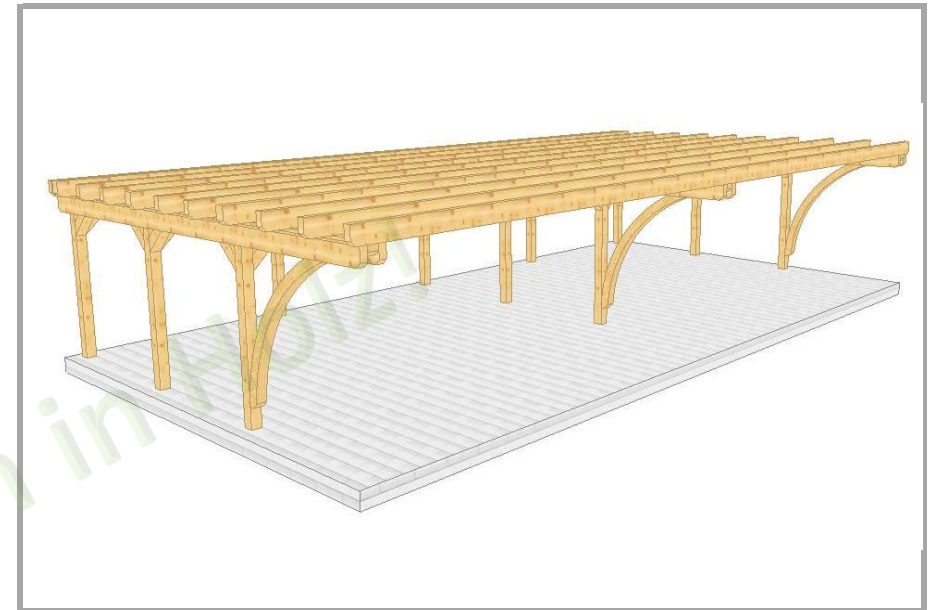
002 3 Vierfach Carport mit Flachdach und 3-Bogenstützen
