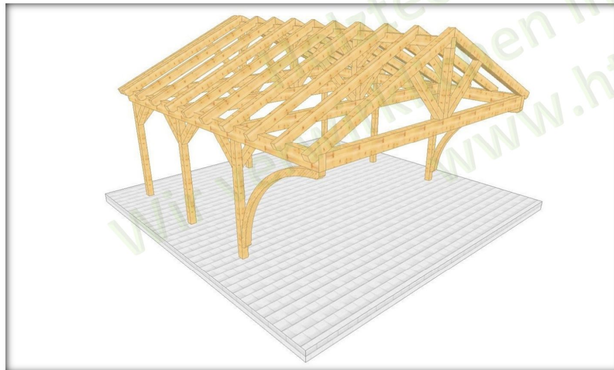
003 3 Doppelcarport mit Bogenstützen
