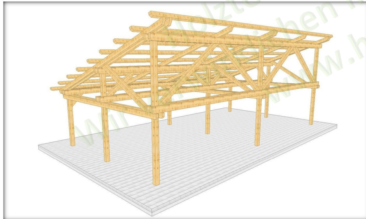
002 3 Solarport Mehrfachcarport
