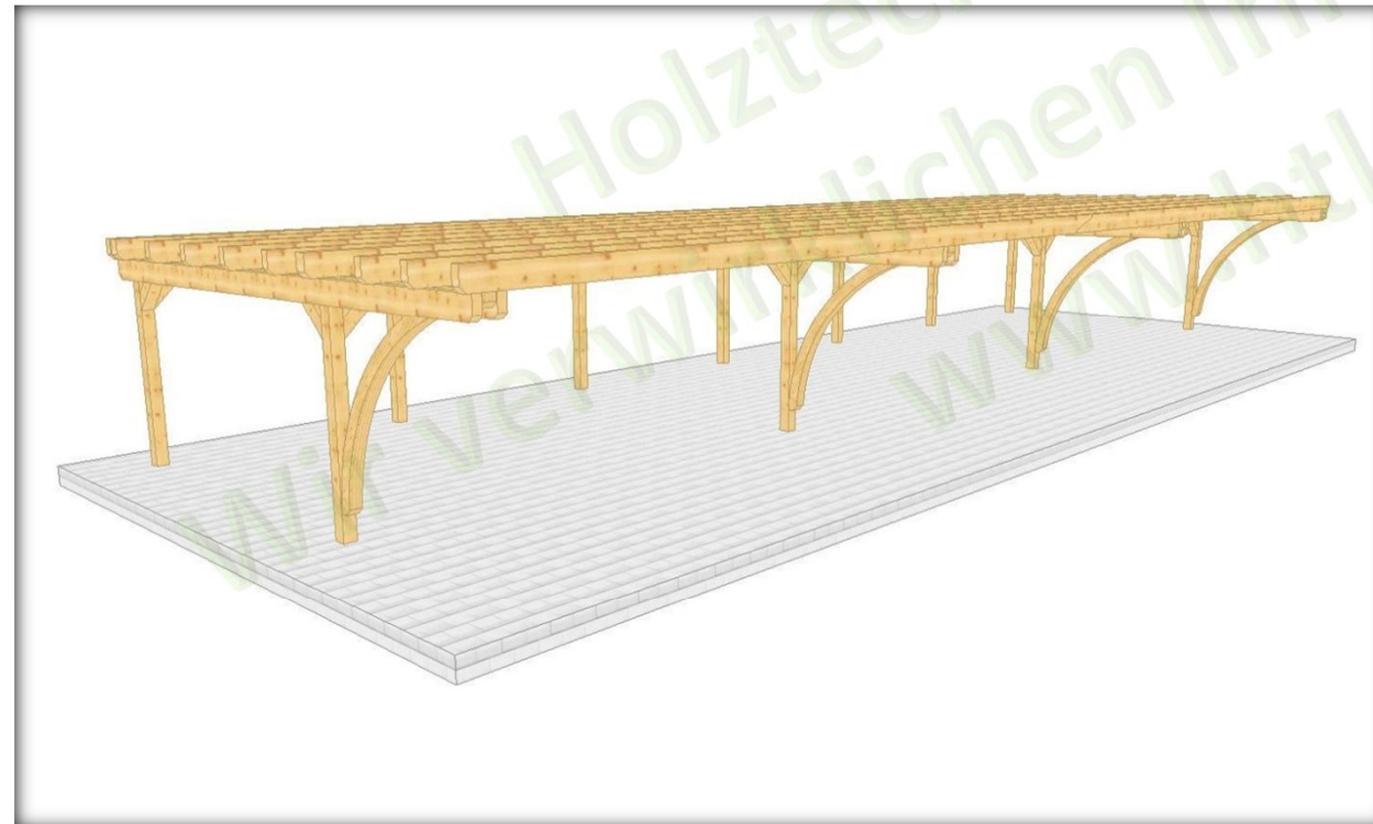
002 3 Reihencarport mit Bogenstützen
