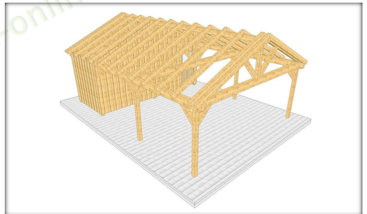
004 3 Doppelcarport mit Schuppen hinten
