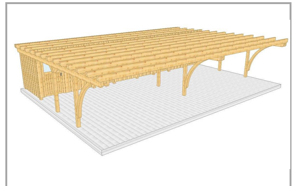
004 3 Vierfach Carport mit Flachdach, 3-Bogenstützen und Abstellraum
