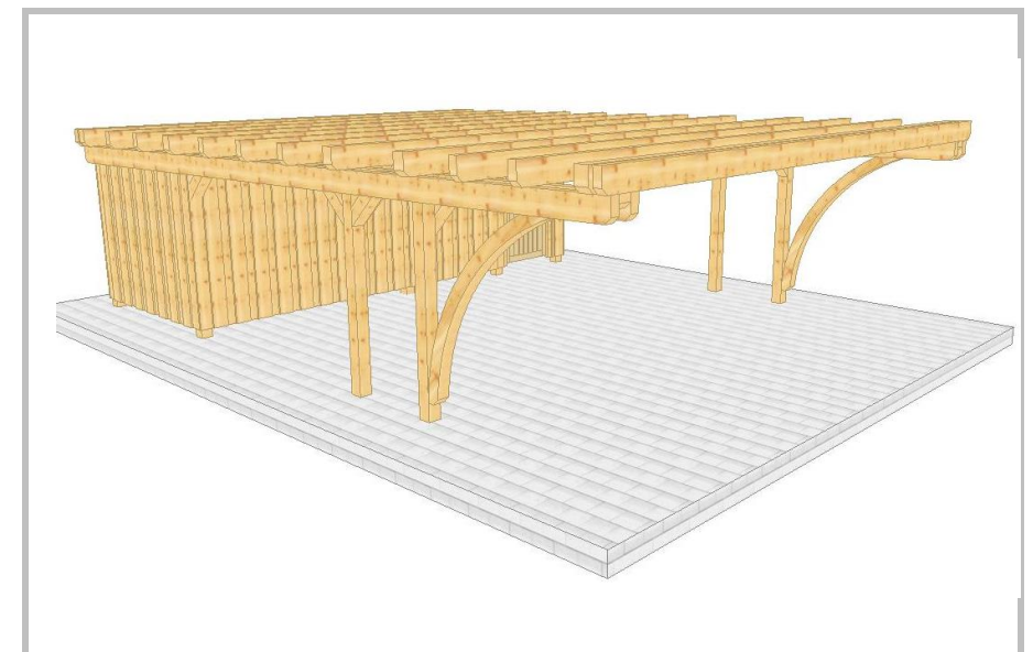
004 3 Doppelcarport mit 2-Bogenstützen und Schuppen, Flachdach
