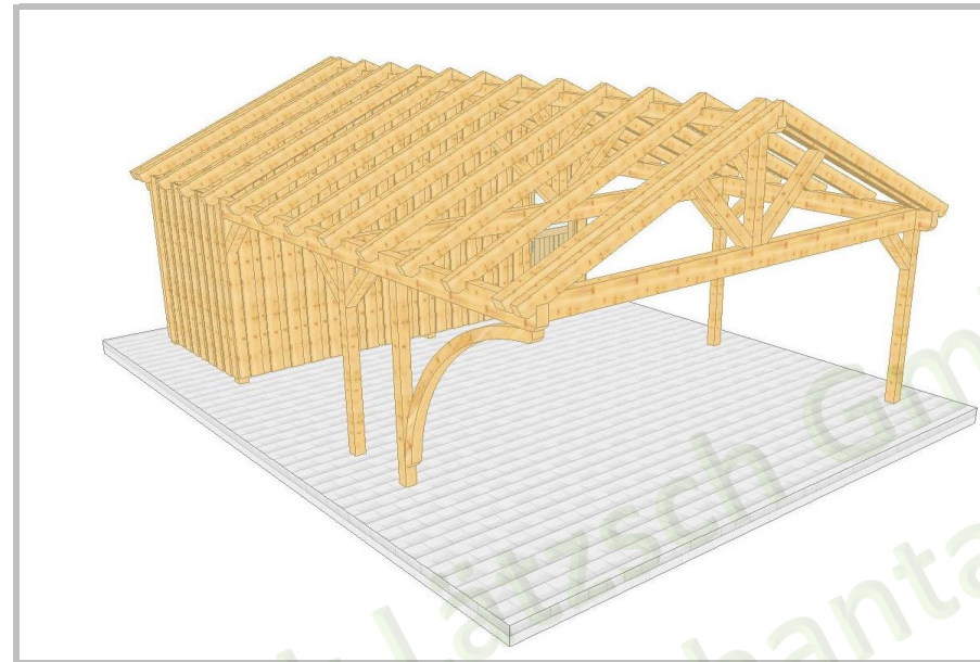
001 3 Doppelcarport mit 1-Bogenstütze und Schuppen, Satteldach
