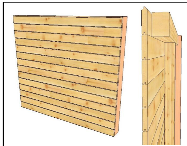
01.1.1 Fichte Faserbrett, waagrecht Fichte Faserbrett 22,5 mm >> Sichtqualität außen, gehobelt Ober- und Untergurt KVH 8 x 12 cm senkrechte 8 x 8 cm
