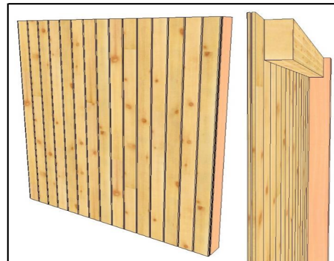
01.1.2 Fichte Faserbrett, senkrecht Fichte Faserbrett 22,5 mm >> Sichtqualität außen, gehobelt Ober- und Untergurt KVH 8 x 12 cm
