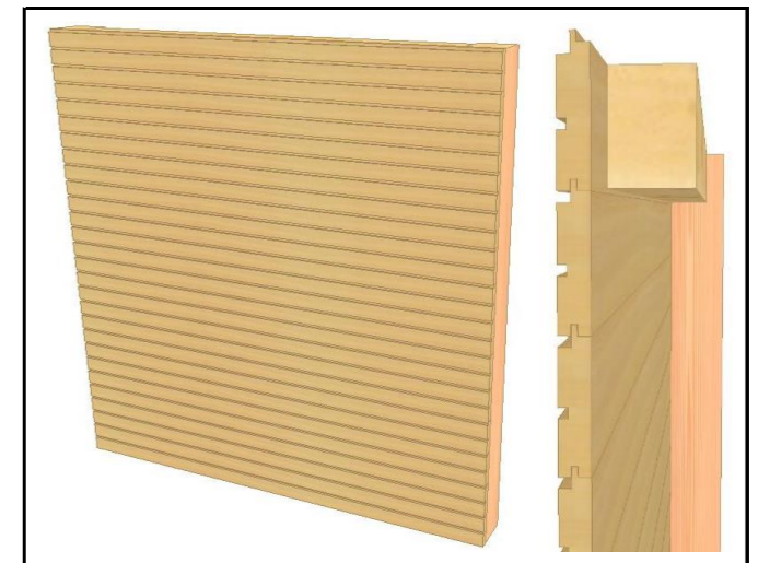
01.1.4 Rhombusschalung, geschlossen vor den Stützen montiert sib. Lärche 27 x 144 mm / Lücke 15 mm >> Sichtqualität, gehobelt Ober- und Untergurt KVH 8 x 12 cm senkrechte 8 x 8 cm
