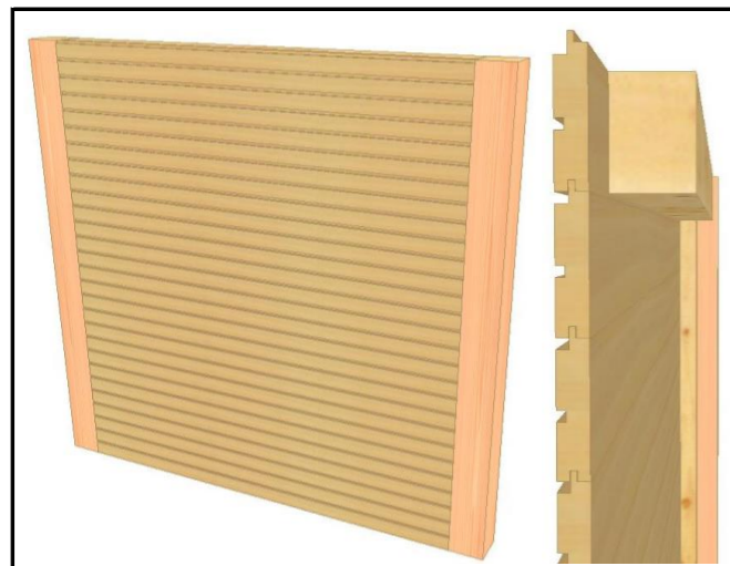
01.1.5 Rhombusschalung, geschlossen zwischen den Stützen montiert sib. Lärche 27 x 144 mm / Lücke 15 mm >> Sichtqualität, gehobelt Ober- und Untergurt KVH 8 x 12 cm senkrechte 8 x 8 cm
