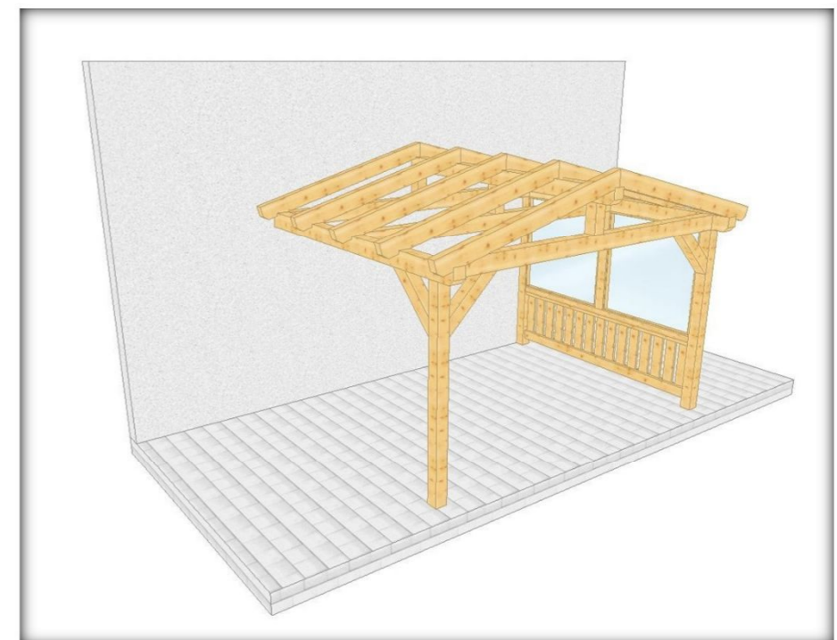
005 3 Überdachung am Haus mit 2 Stützen, Wandverglasung, Geländer
