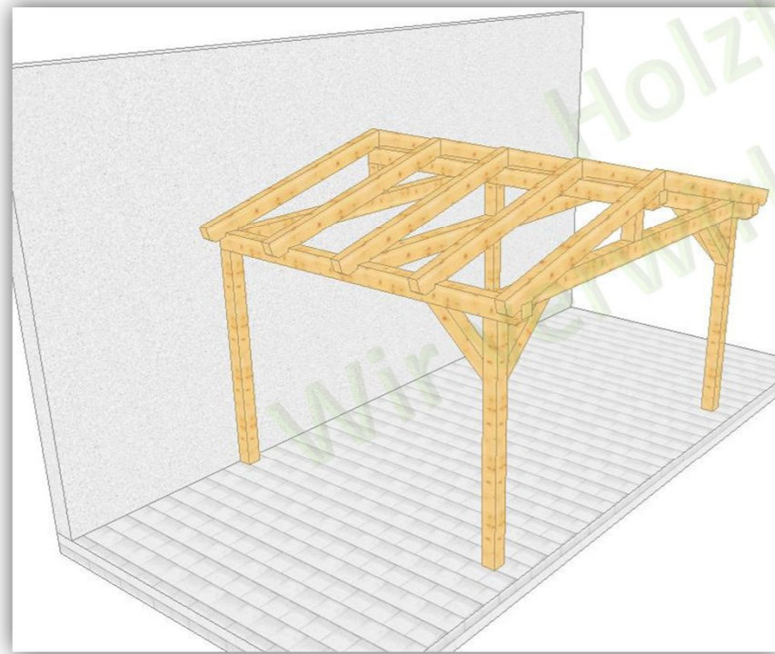
004 3 Überdachung am Haus mit 2 Wandstützen, Satteldach
