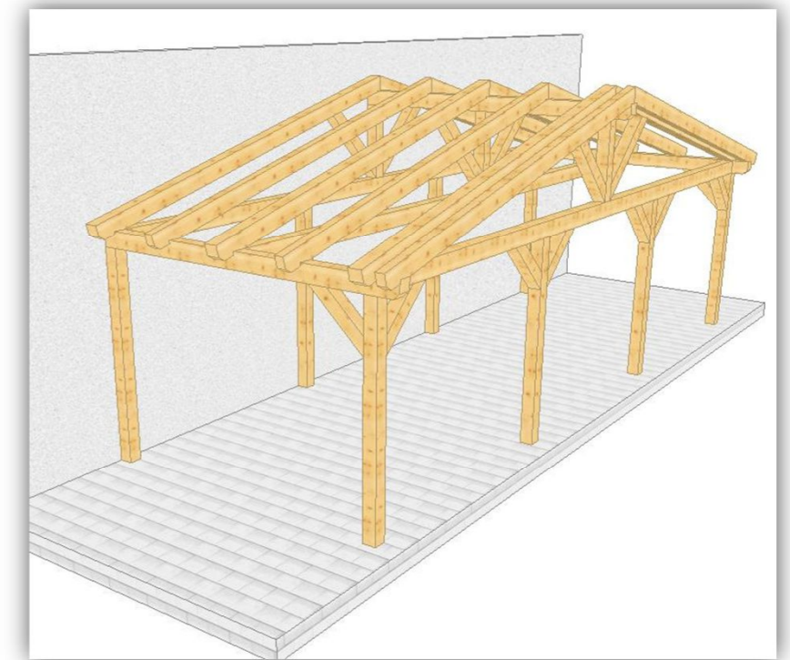
006 3 Überdachung am Haus mit 4 Wandstützen, Satteldach
