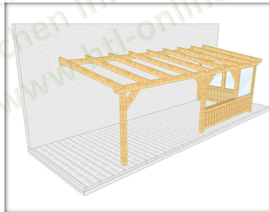
011 3 Überdachung am Haus mit 3 Stützen, Wandverglasung + Geländer
