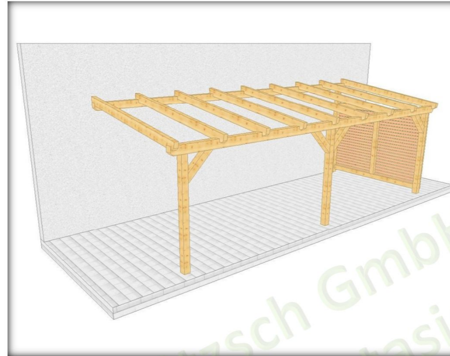
008 3 Überdachung am Haus mit 3 Stützen, mit Wandverschalung
