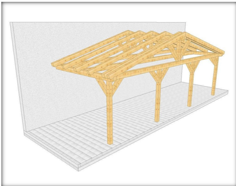
011 3 Überdachung am Haus mit 4 Stützen
