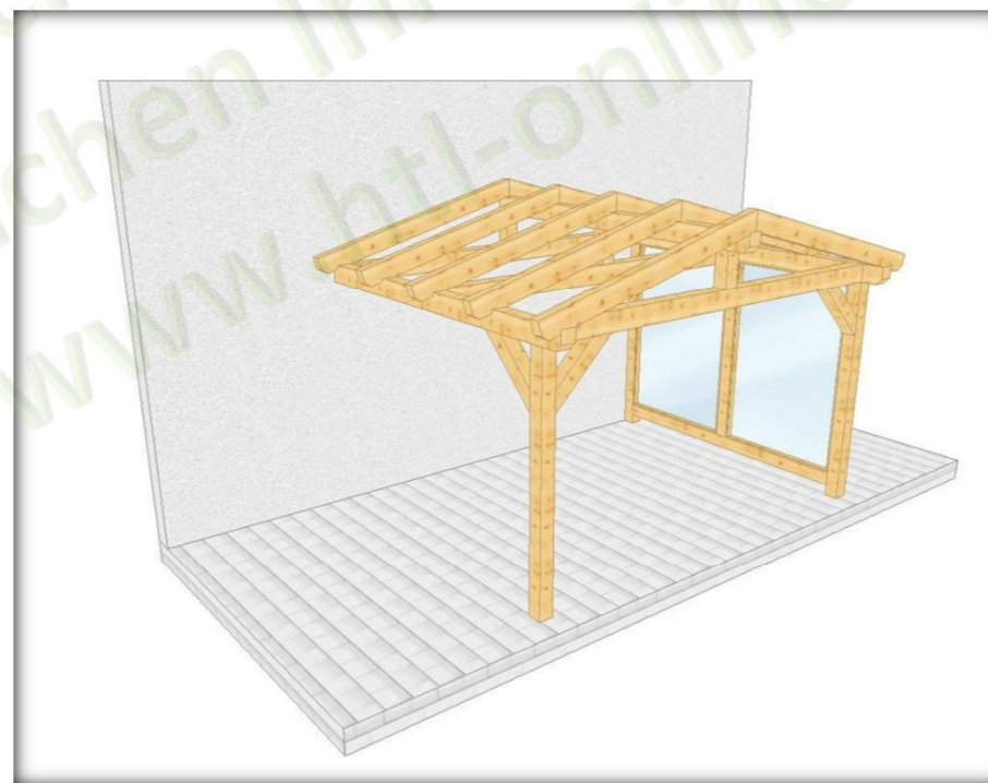
004 3 Überdachung am Haus mit 2 Stützen, mit Wandverglasung
