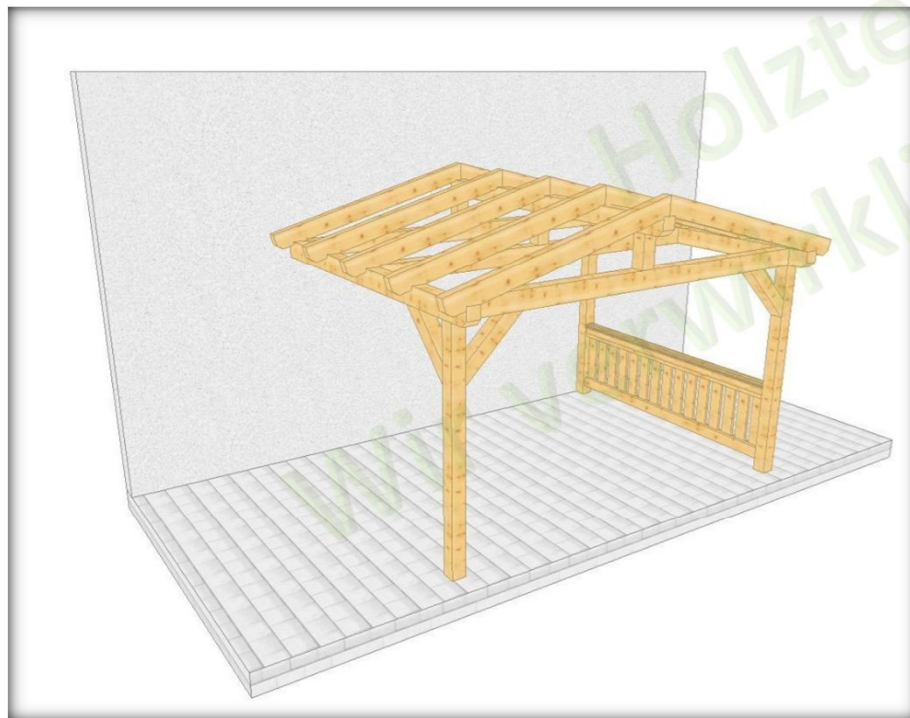
003 3 Überdachung am Haus mit 2 Stützen, mit Geländer
