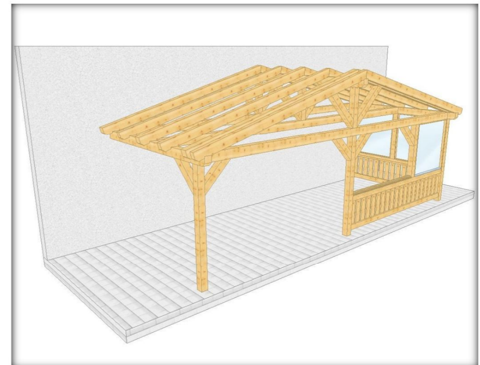
010 3 Überdachung am Haus 3 Stützen, Wandverglasung und Geländer
