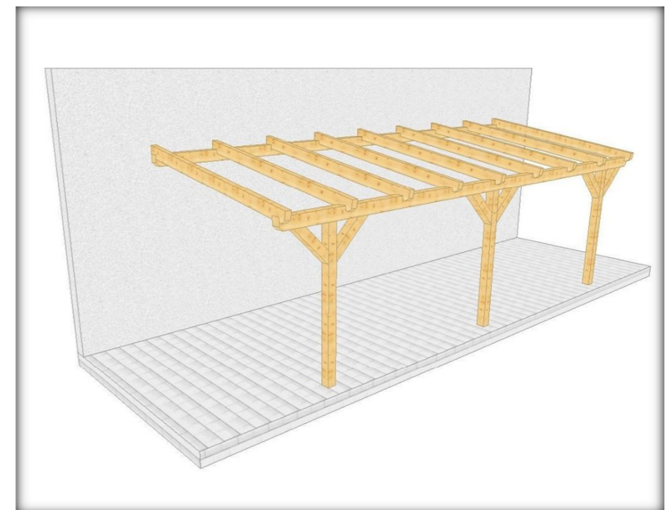
012 3 Überdachung am Haus mit 3 Stützen, eingerückt
