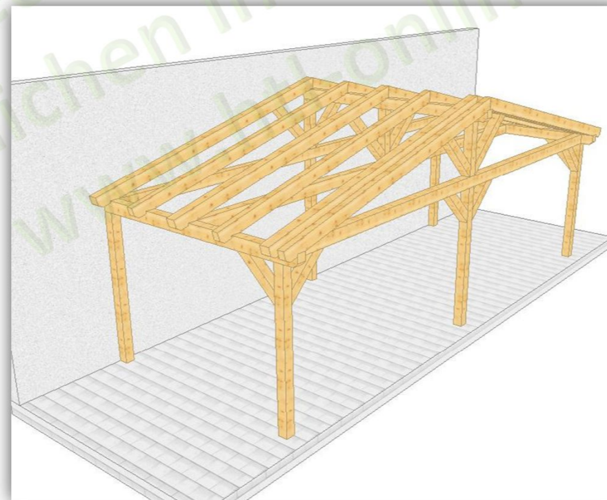
005 3 Überdachung am Haus mit 3 Wandstützen, Satteldach
