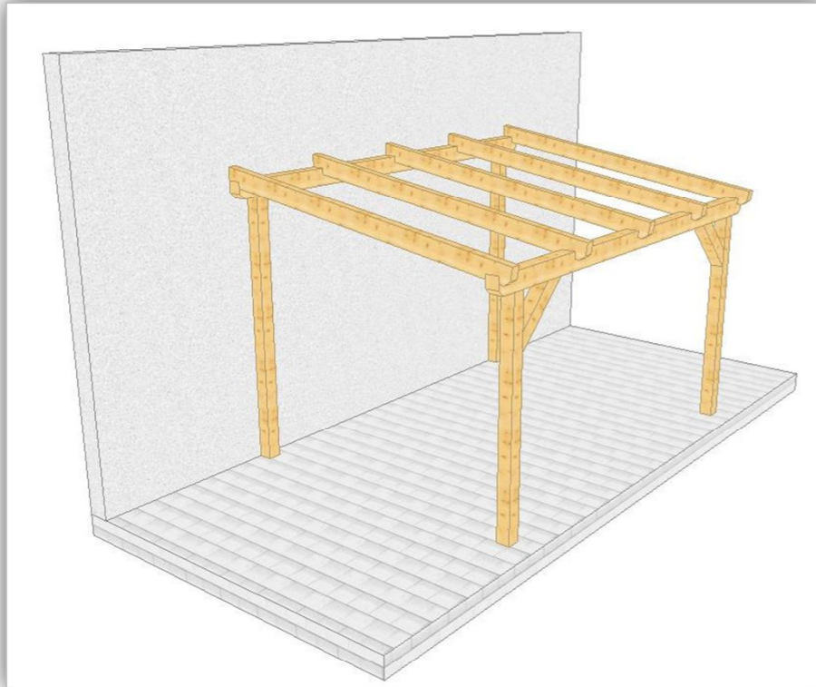
001 3 Überdachung am Haus mit 2 Wandstützen, Pulldach
