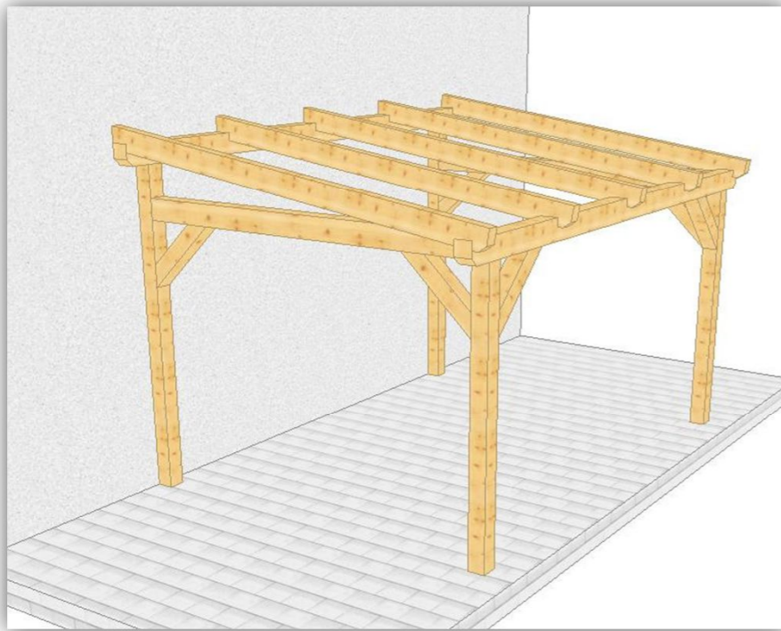
1 Überdachung freistehend am Haus verankert 2 Stützen
