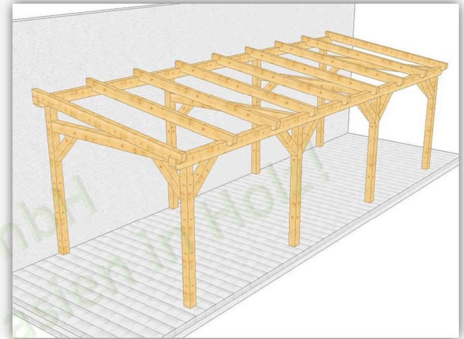
3 Überdachung freistehend am Haus verankert 4 Stützen
