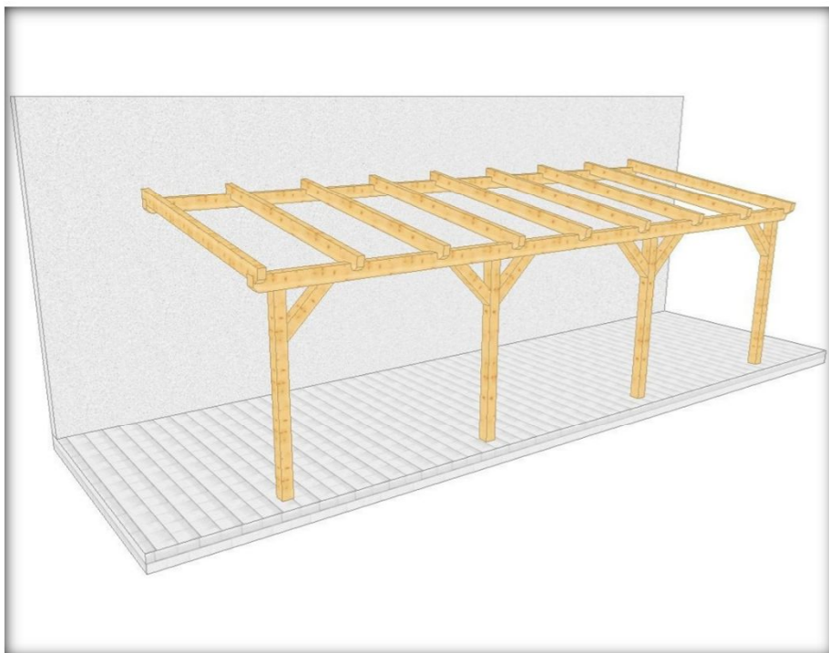
013 3 Überdachung am Haus mit 4 Stützen
