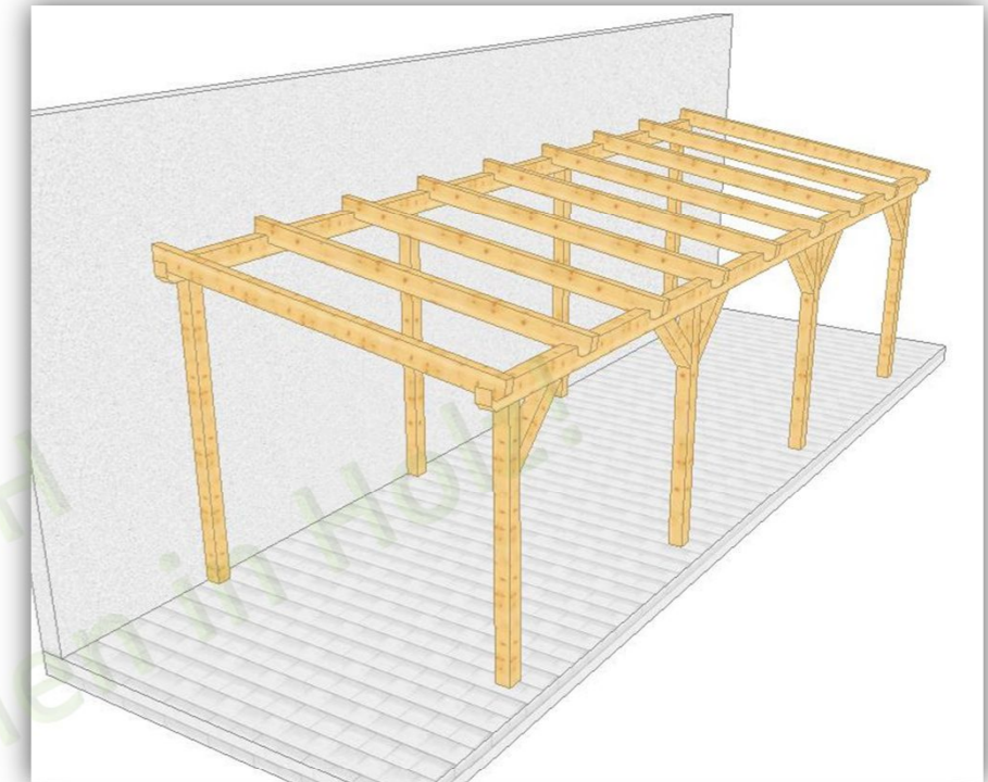
003 3 Überdachung am Haus mit 4 Wandstützen, Pulldach
