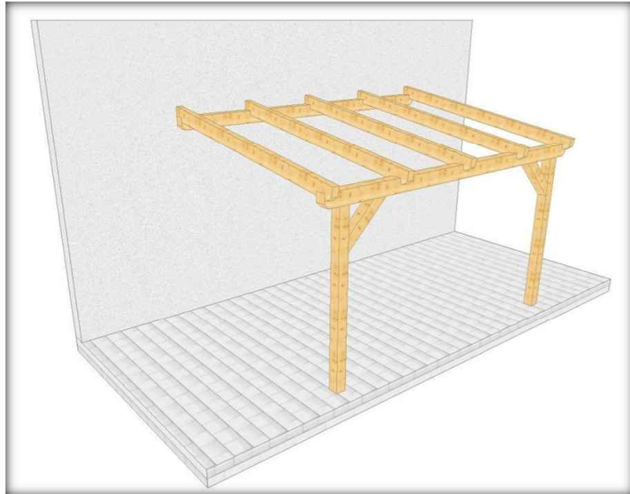
001 3 Überdachung am Haus mit 2 Stützen
