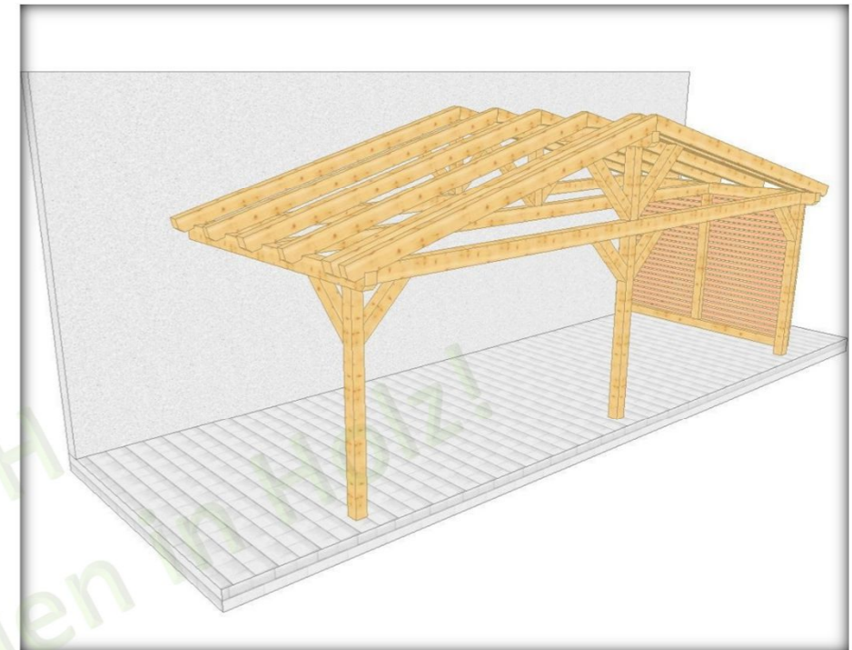
007 3 Überdachung am Haus mit 3 Stützen, mit Wandverschalung
