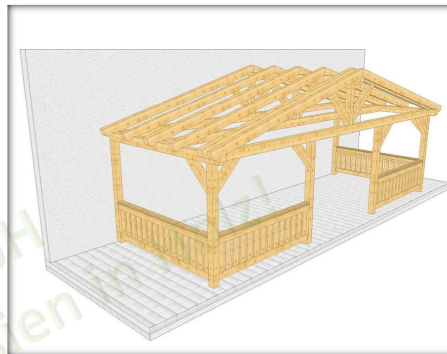
013 3 Überdachung am Haus mit 4 Stützen, mit Geländer
