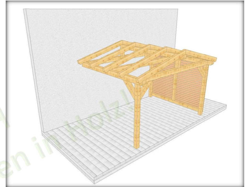
002 3 Überdachung am Haus mit 2 Stützen, mit Wandverschalung
