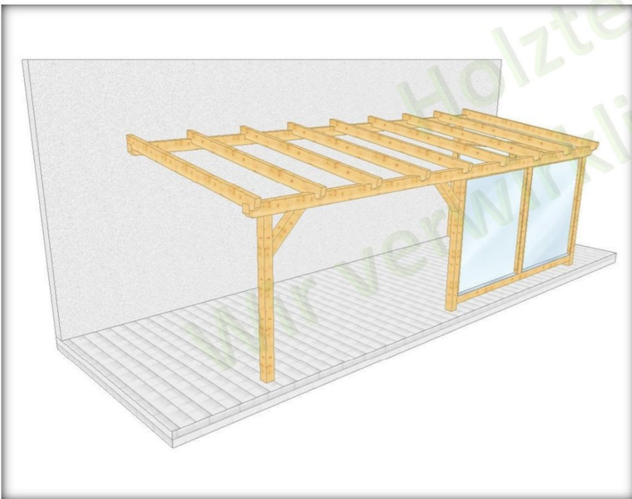
010 3 Überdachung am Haus mit 3 Stützen, mit Wandverglasung
