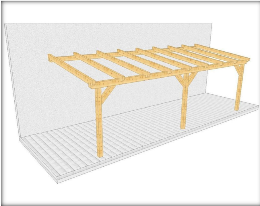
007 3 Überdachung am Haus mit 3 Stützen
