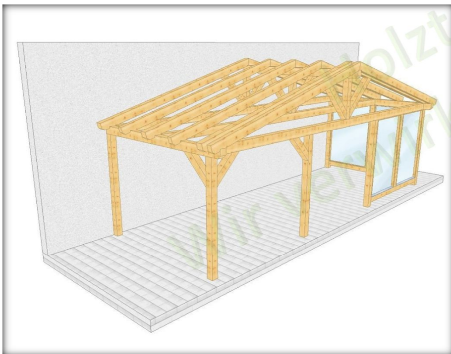
014 3 Überdachung am Haus mit 4 Stützen, mit Wandverglasung
