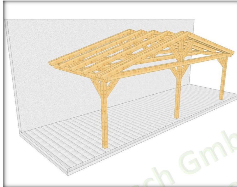
006 3 Überdachung am Haus mit 3 Stützen
