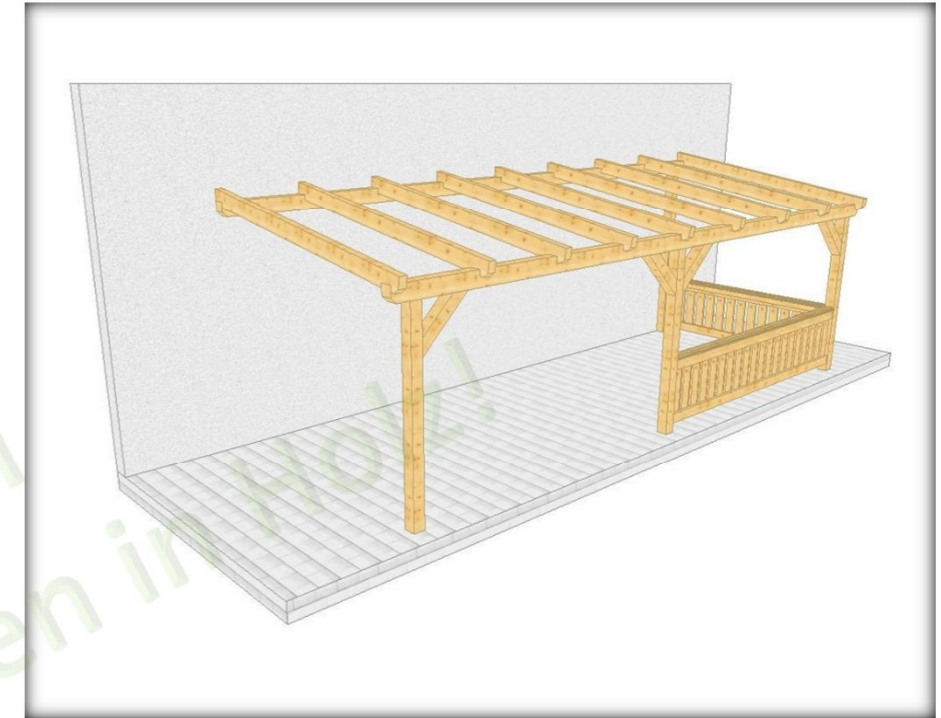
009 3 Überdachung am Haus mit 3 Stützen, mit Geländer
