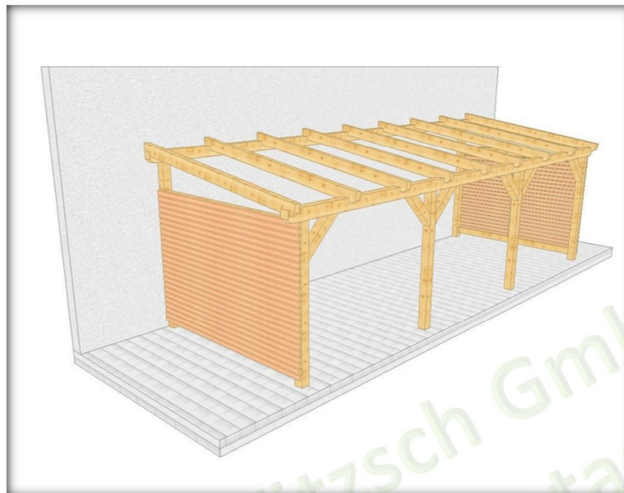
014 3 Überdachung am Haus mit 4 Stützen, mit Wandverschalung
