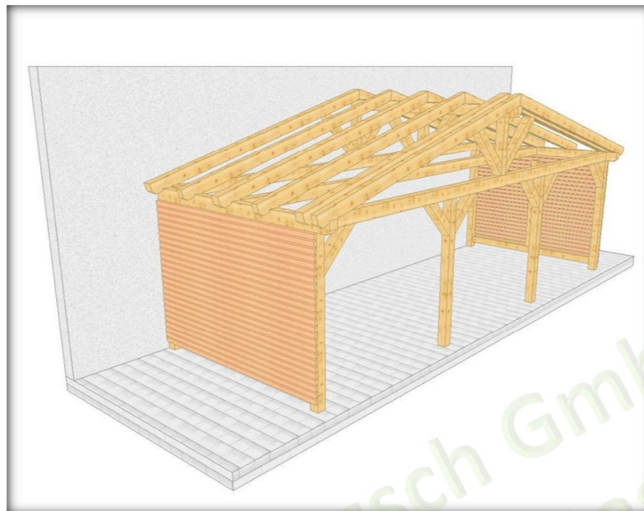
012 3 Überdachung am Haus mit 4 Stützen, mit Wandverschalung
