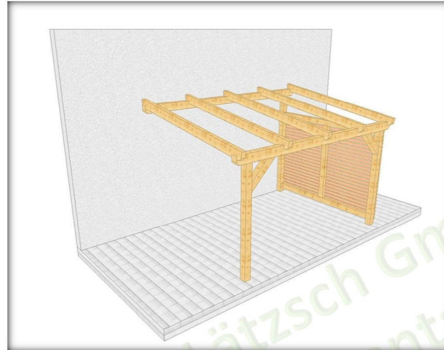
002 3 Überdachung am Haus mit 2 Stützen, mit Wandverschalung
