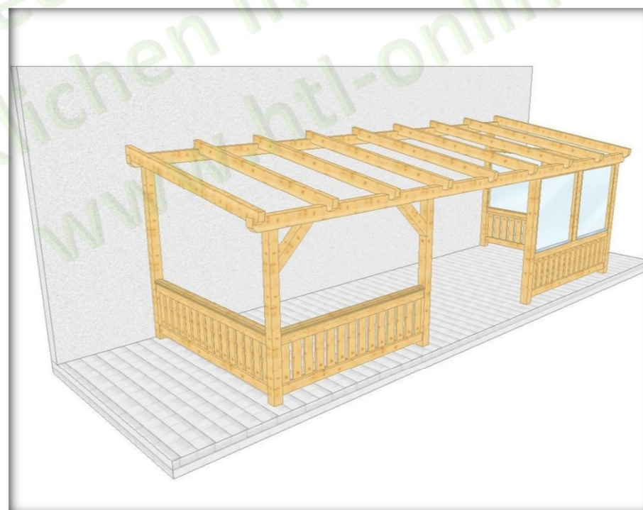
017 3 Überdachung am Haus mit 4 Stützen, Wandverglasung + Geländer
