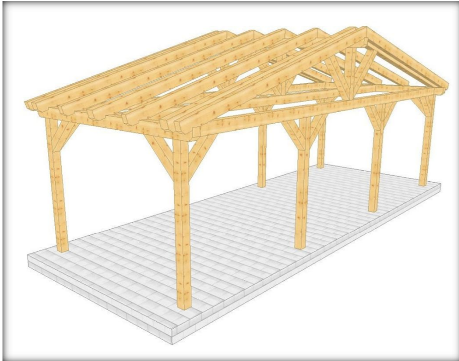
011 3 Überdachung freistehend mit 8 Stützen, Satteldach
