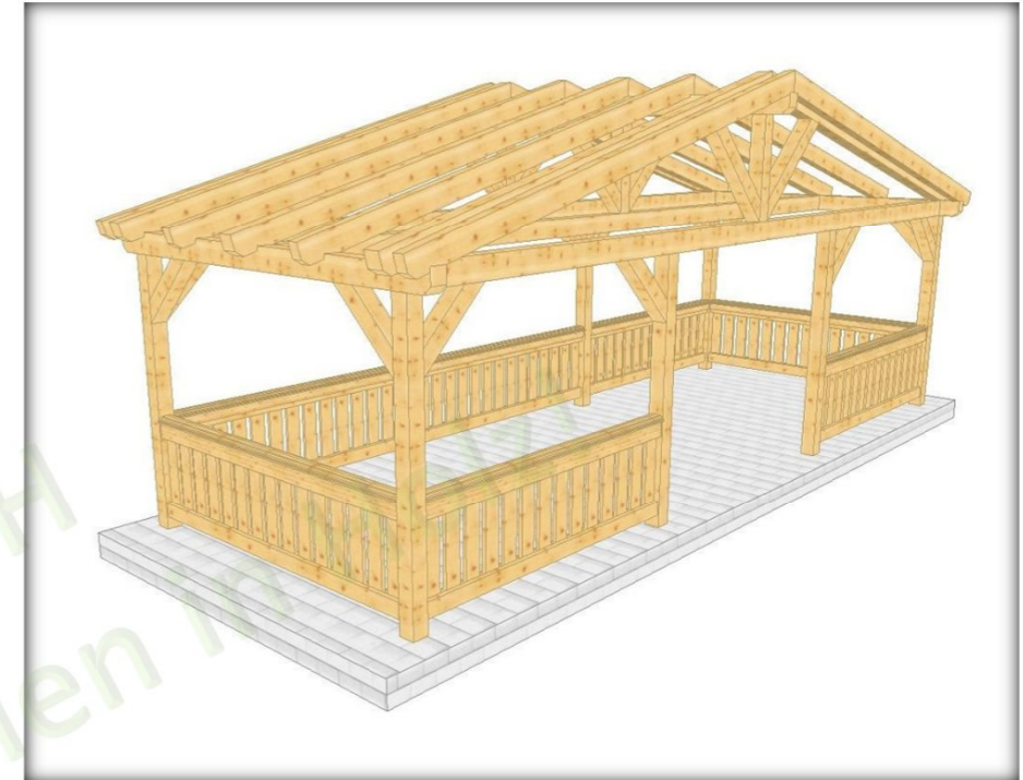
013 3 Überdachung freistehend mit 8 Stützen, mit Geländer, Satteldach
