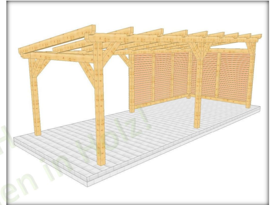
007 3 Überdachung freistehend 6 Stützen, Wandverschalung, Pultdach
