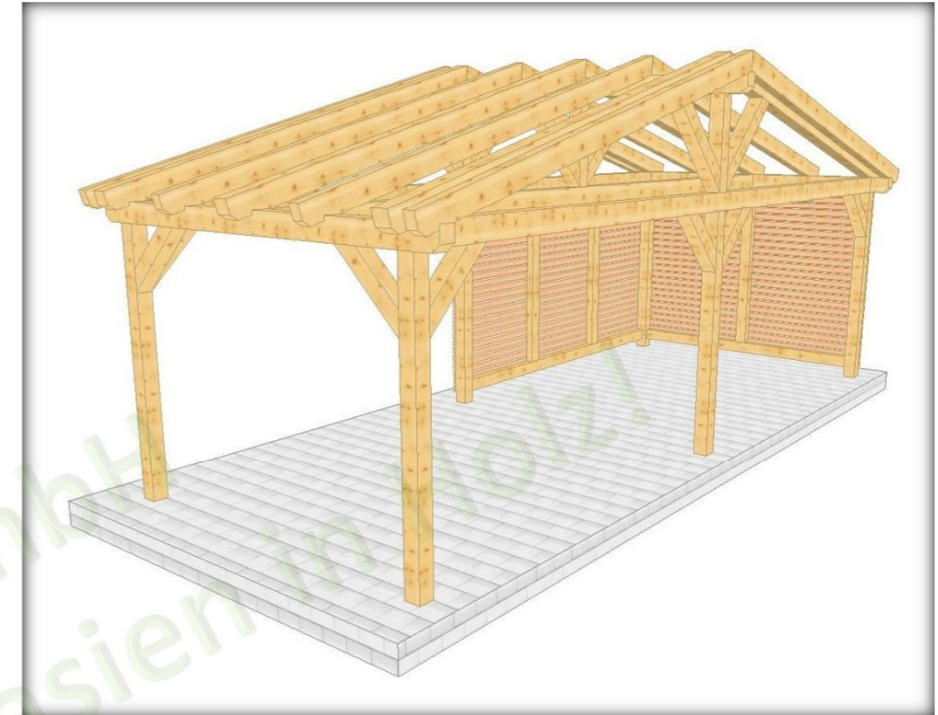
007 3 Überdachung frei 6 Stützen, Wandverschalung, Satteldach
