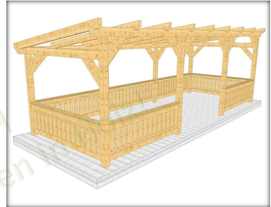
013 3 Überdachung freistehend mit 8 Stützen, mit Geländer, Pultdach
