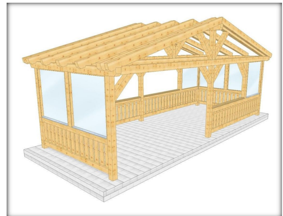
010 3 Überdachung frei 6 Stützen, Verglasung, Geländer, Satteldach
