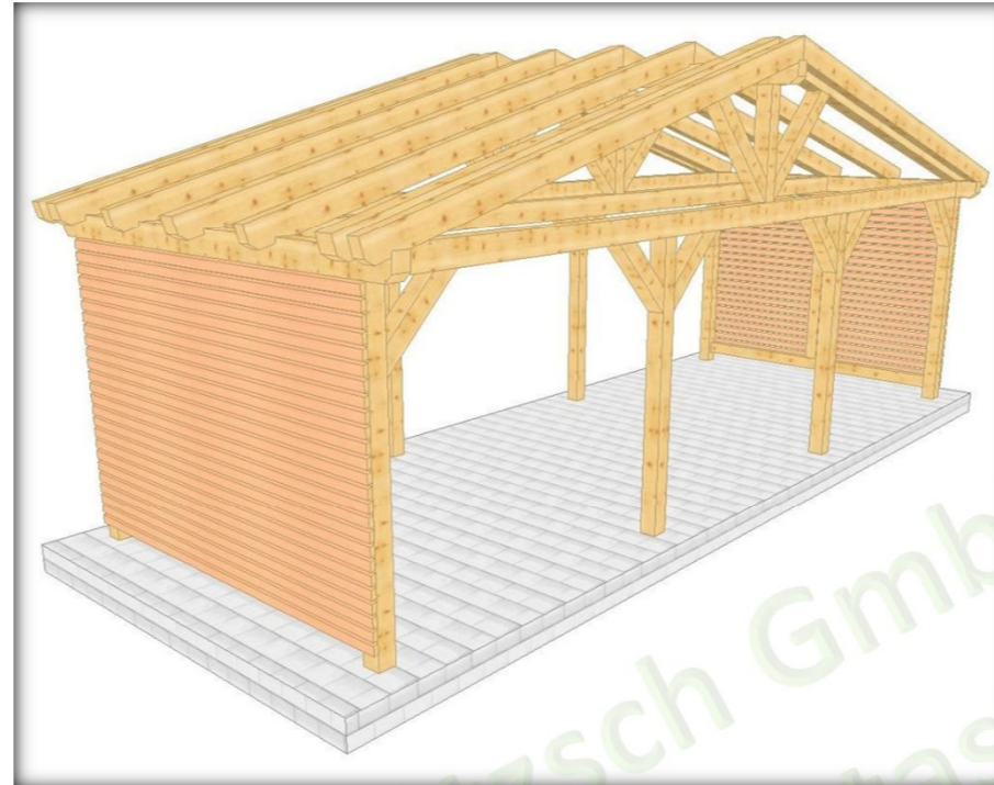
012 3 Überdachung frei 8 Stützen, Wandverschalung, Satteldach
