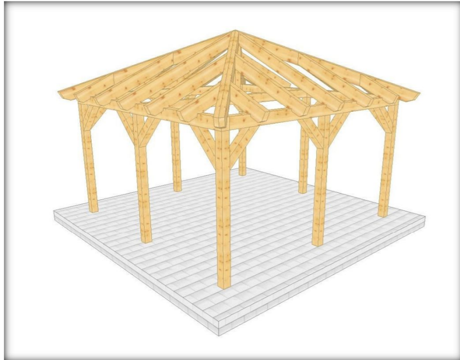
006 3 Überdachung freistehend mit 8 Stützen, Walmdach
