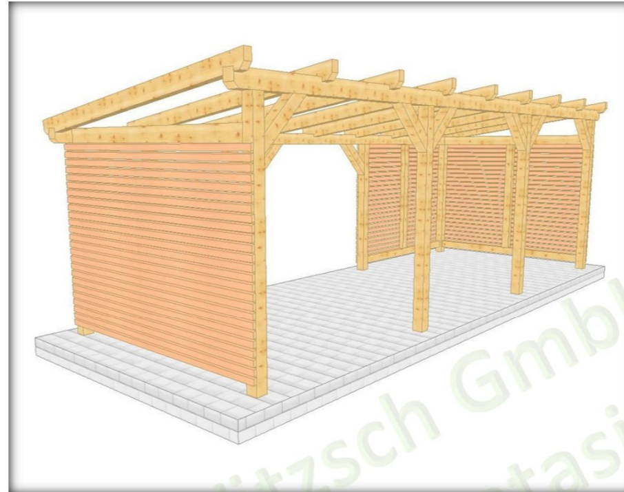
012 3 Überdachung freistehend 8 Stützen, Wandverschalung, Pultdach
