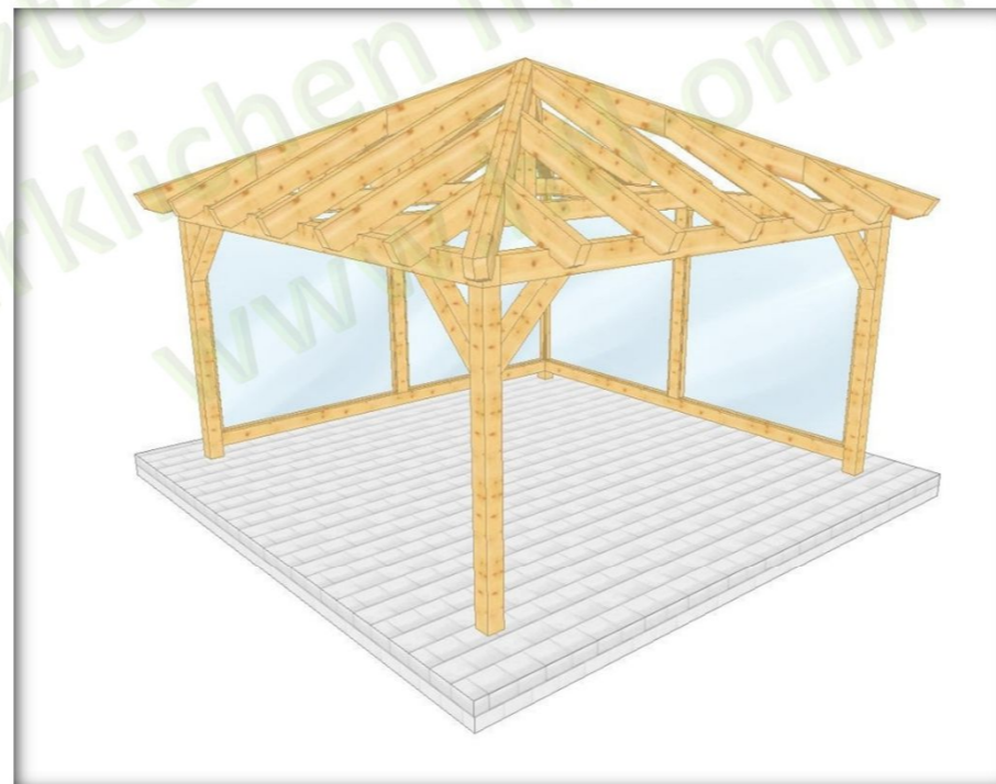
004 3 Überdachung frei mit 4 Stützen, Wandverglasung, Walmdach
