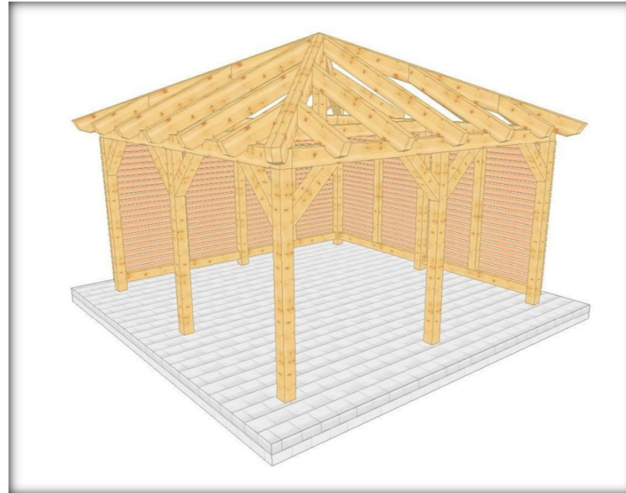
007 3 Überdachung freistehend 8 Stützen, Verschalung, Walmdach
