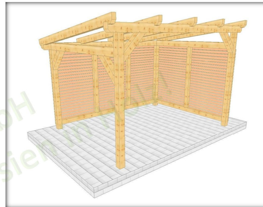
002 3 Überdachung freistehend 4 Stützen, Wandverschalung, Pultdach
